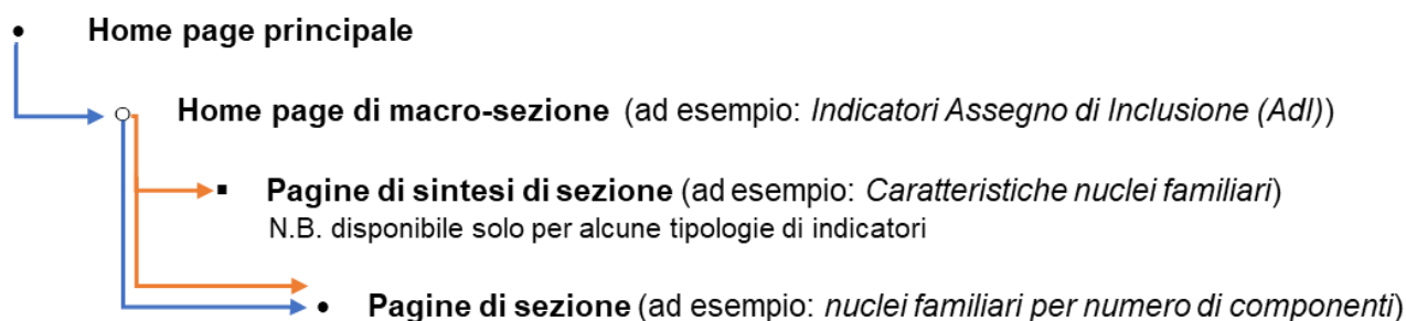
Figura 1 - Gerarchia dashboard
